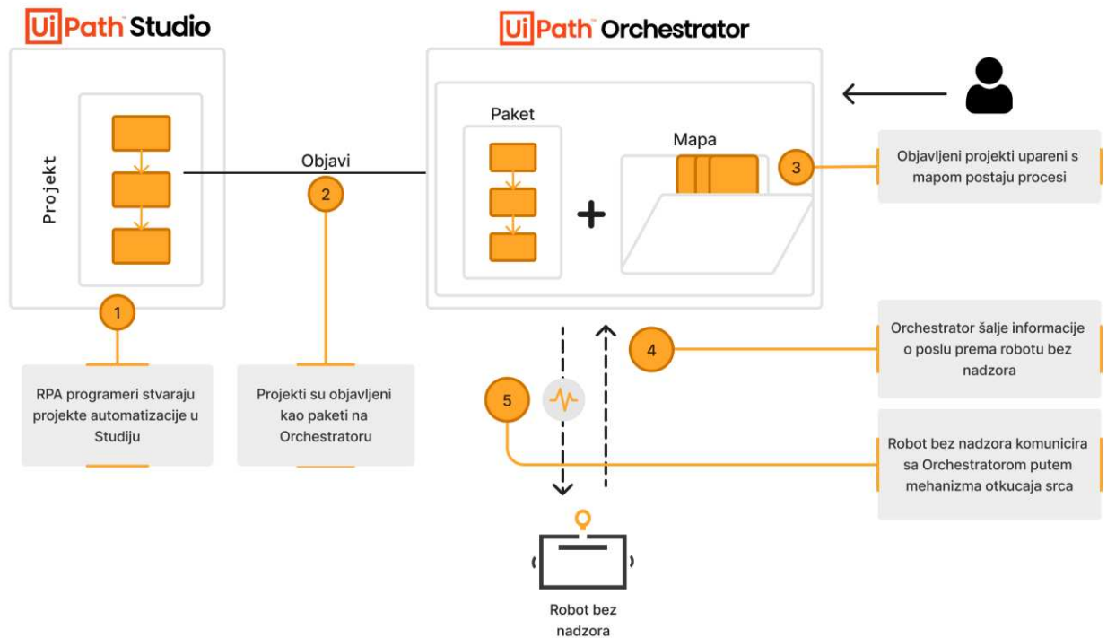
Slika 10. Veza UiPath komponenata (UiPath Forum, 2023)
