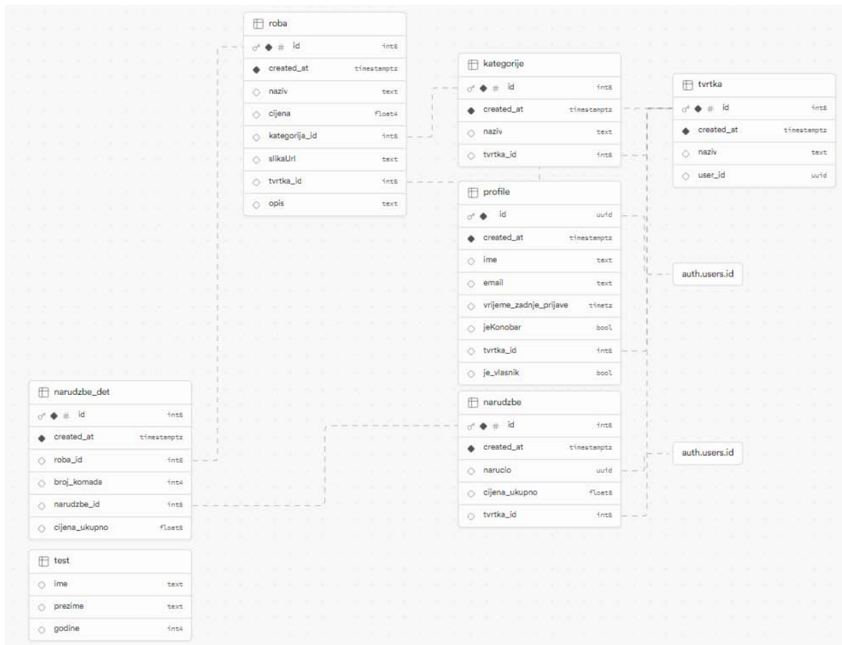
Slika 4. Schema Visualizer
